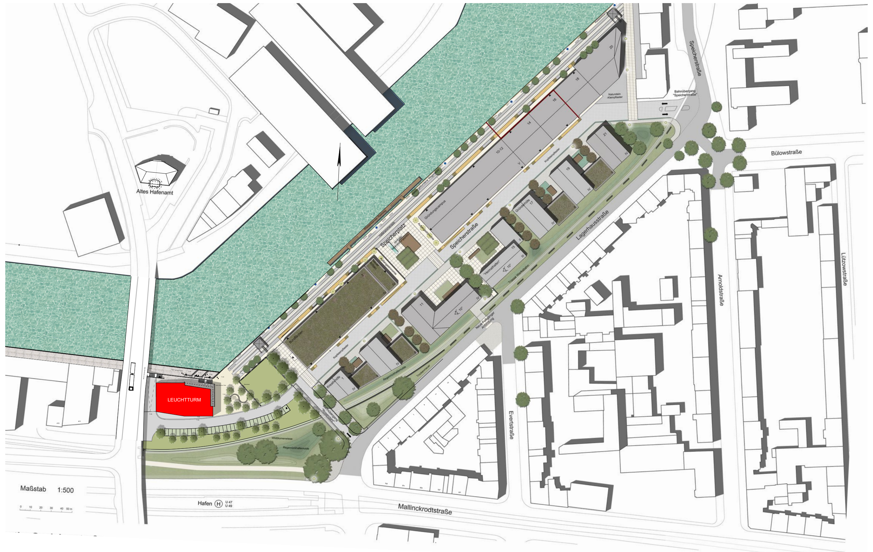
Lageplan (1.OG) M 1: 1500
